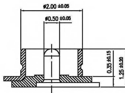
SEC. A-A
