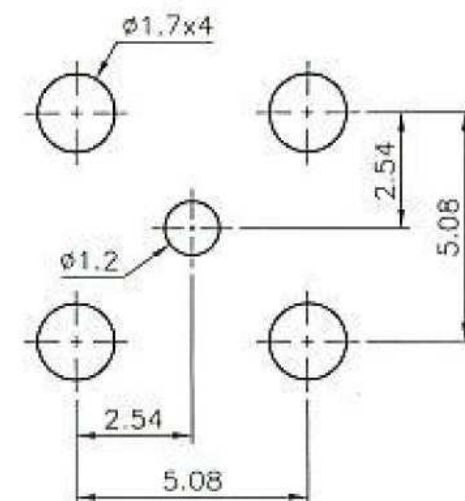
P.C.B. LAYOUT
